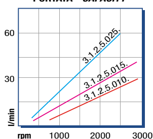
PORTATA - CAPACITY
